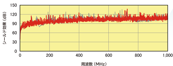
Y-Shield YS-FP シールド性能
